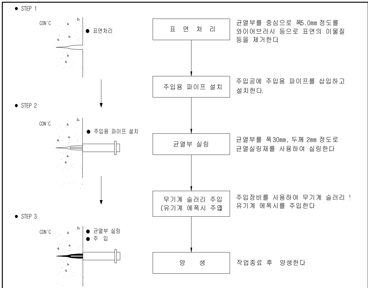
【그림 6.2】 균열 보수공법 개요도
